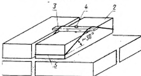
Схема захвата кирпича, подготовленного к испытанию
