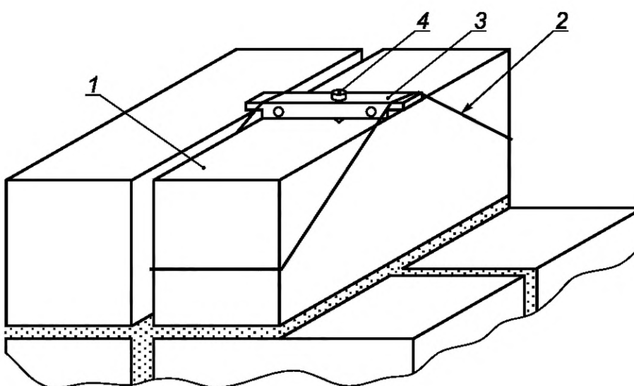
б) схема захвата природного камня
