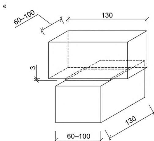
а) Образец из половинок кирпича».
