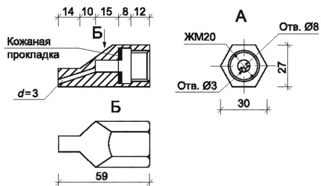
Рисунок Д.4 — Переходник (позиция 12 рисунка 1)
