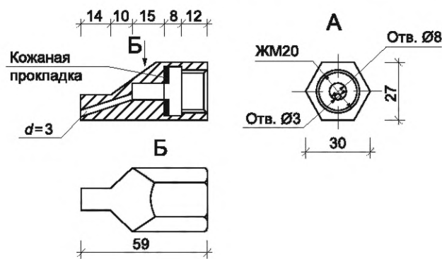
Рисунок Д.4 — Переходник (позиция 12 рисунка 1)
