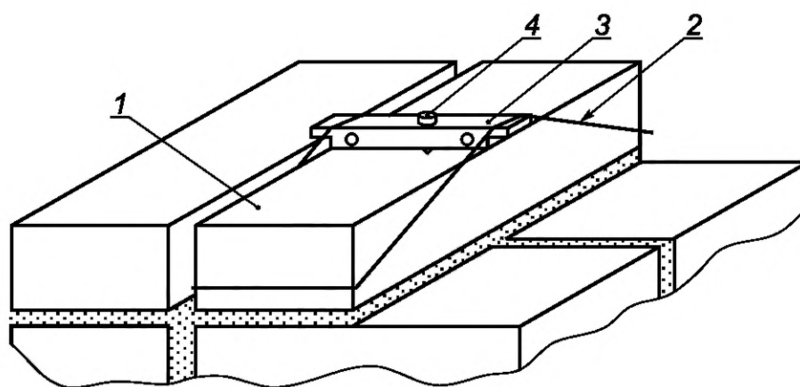
а) схема захвата кирпича
