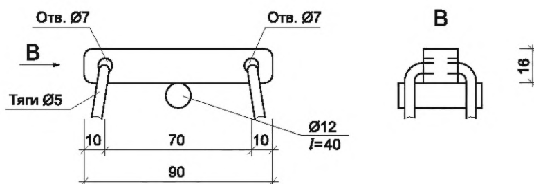
Рисунок Д.3 — Траверса (позиция 9 рисунка 1)
