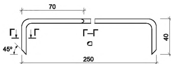
Рисунок Д.5 — Угловой скребок
