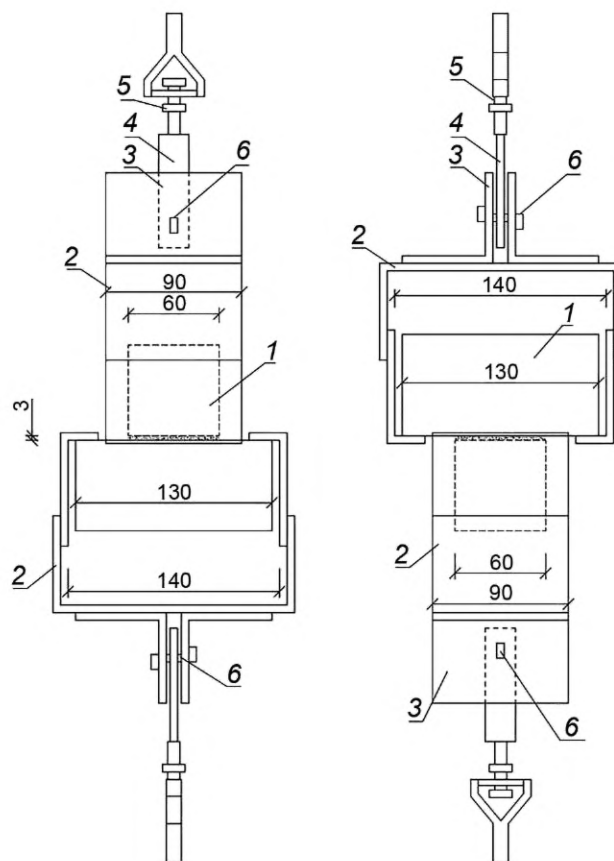
1 — испытуемый образец из камня; 2 — металлический захват; 3 — уголки 60×60×6 мм; 4 — металлическая пластина 20×90×6 мм; 5 — шарнир; 6 — шпилька
