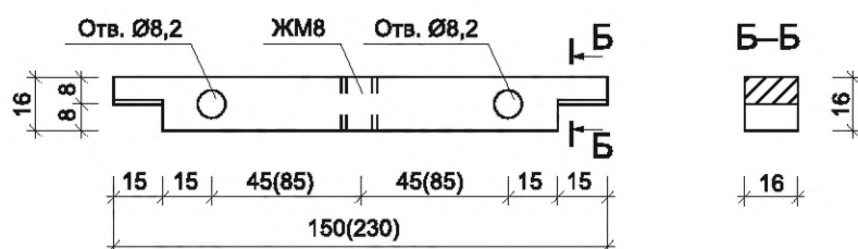
Рисунок Д.2 — Перекладина (позиция 3 рисунка 1)
