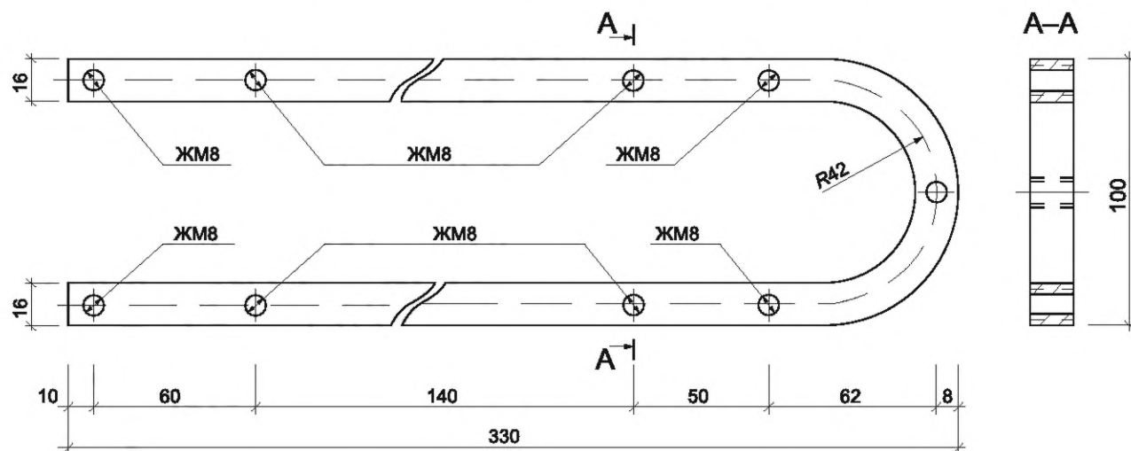
Рисунок Д.1 — Рама (позиция 11 рисунка 1)
