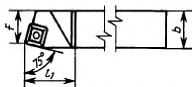
Левый резец
