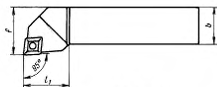
Левый резец
