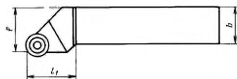
Левый резец
