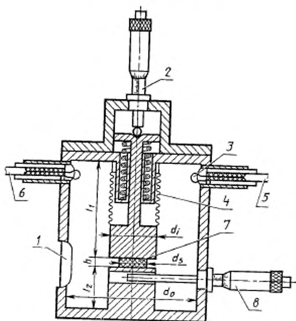
1 — корпус; 2 — главный микрометр; 3 — петля связи; 4 — металлическая гармоника; 5 — к генератору; 6 — к детектору; 7 — образец; 8 — боковой микрометр
