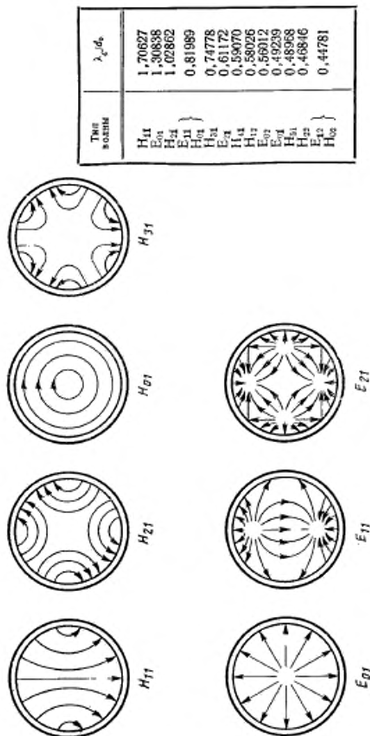
Мгновенная конфигурация поля и выключающая длина волны некоторых типов волн низкой частоты цилиндрического резонатора
