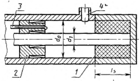
1 — образец; 2 — скользящий плунжер; 3 — от генератора; 4 — к детектору
