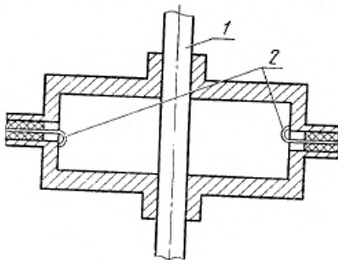
Закрытый резонатор с волной типа E=TM_{010}
