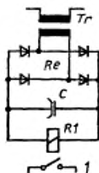
I — выключатель, питание (I5 по черт. 2а); Re — выпрямитель; Tr — трансформатор (обмотка 300/300 витков); R1 — реле (2500 Ом/1100 витков); C — конденсатор (200 мкФ)
