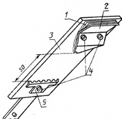
1 — тампон фильтровальной бумаги под верхним электродом; 2 — верхний электрод; 3 — испытуемый образец; 4 — 3 винта 4×20 мм, 6 шайбы, 3 гайки — все из нержавеющей стали; 5 — нижний электрод
