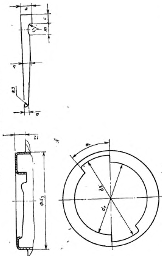
Размеры горловины с байонетным замком
