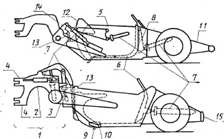
1 — тяговая рама; 2 — хобот; 3 — упругая тяга; 4 — кронштейн поворотного шкворня; 5 — ковш; 6 — задняя стенка ковша; 7 — гидроцилиндр; 8 — рычаг задней стенки; 9 — режущий нож; 10 — подрезной нож; 11 — буферная рама; 12 — заслонка; 13 — тяга заслонки или ковша; 14 — рычаг заслонки или ковша; 15 — буфер
