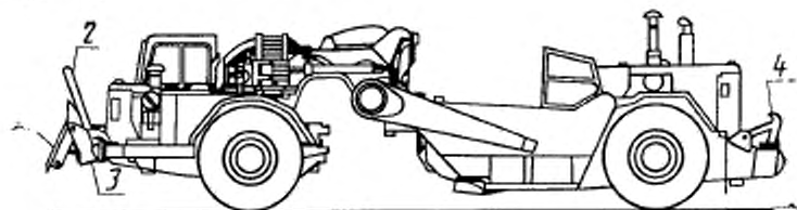
1 — передняя толкающая плита; 2 — скоба; 3 — охваты скобы; 4 — крюк
