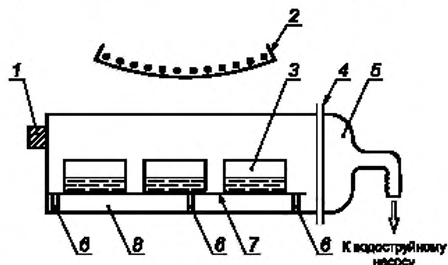
1 — пробка; 2 — нагреватель мощностью 150 в, обеспечивающий плавное регулирование температуры нагрева; 3 — чаши с пробой; 4 — плоский шлиф, закрепляемый зажимом; 5 — колпак сосуда; 6 — кварцевые ножки; 7 — подставка для чаш из кварца; 8 — сосуд из кварцевого стекла
