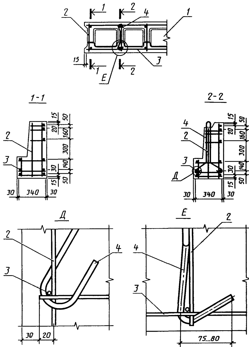
План блока типа БЧ с четвертью поперечного сечения № 2
