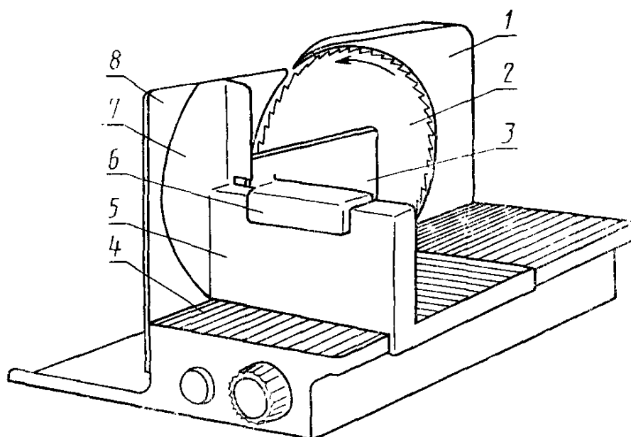
1—защита ножа; 2—нож; 3—держатель ломтика. 4—суппорт; 5—подающая доска; 6—опора для руки, 7—защита большого пальца, 8—пластина, регулирующая толщину нарезаемых лом- тей.
