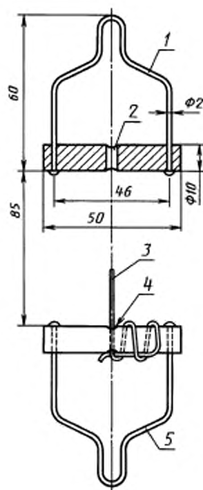
1 — неподвижный хомут, 2 — отверстие диаметром 4 мм с закругленными краями; 3 — образец; 4 — отверстие; 5 — подвижный хомут
