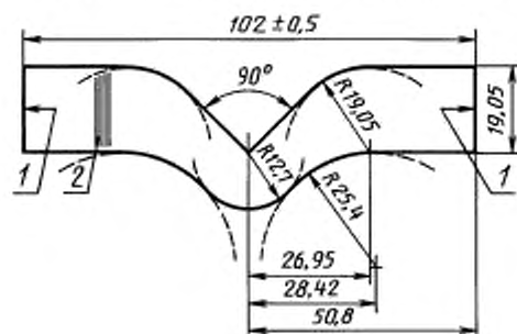
Матрица для испытания прочности на разрыв по п. 21.12
