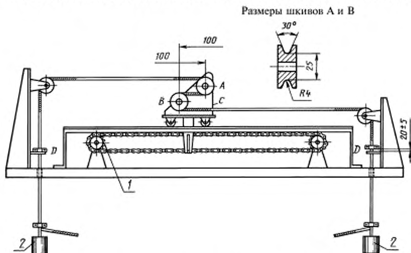
A, B — шкивы; C — салазки, D — сдерживающие зажимы; 1 — звездочка ( d_{cp} = 88,9 мм, z = 20 , шаг 12,7 мм); 2 — груз массой 0,25 кг
