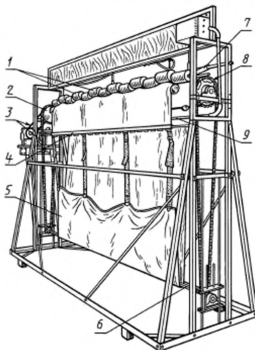
1 — заблокированные валики; 2 — самовыравнивающиеся подшипники; 3 — приводная шестерня; 4 — зажимная балка; 5 — испытываемое одеяло; 6 — балка квадратного сечения; 7 — рычаги валиков; 8 — звездочка; 9 — подвижная балка
