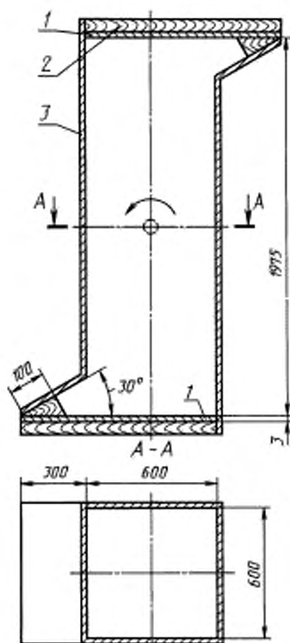
1 — стальная плита; 2 — деревянная опора; 3 — гладкие металлические стороны
