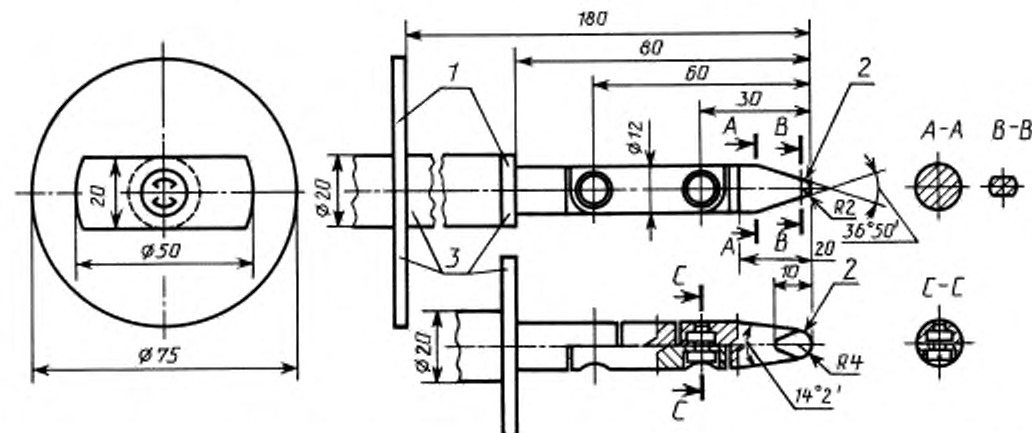
Стандартный испытательный палец для испытания по п. 8.1
