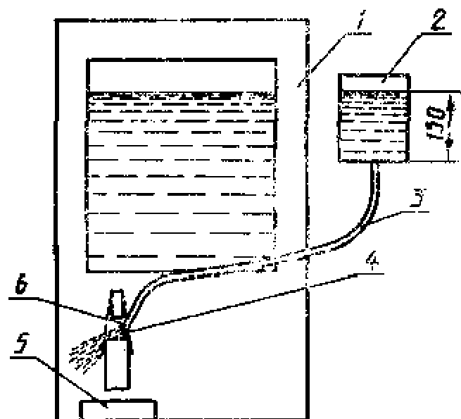
Оборудование для испытания на повреждение соединений
