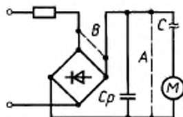
Последовательная цепь
