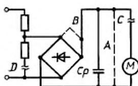
Параллельная цепь
