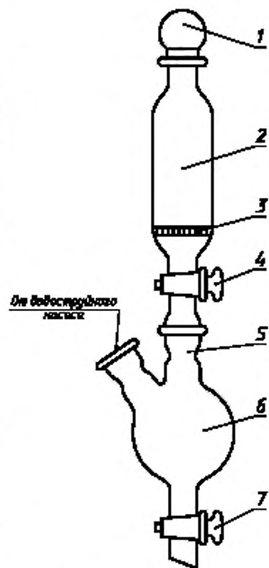
1 — пробка (притертая); 2 — фильтрующая делительная воронка; 3 — впаиваемый стеклянный фильтр № 2 или 3; 4, 7 — сливные краны; 5 — соединительный шлиф; 6 — приемник экстракта
