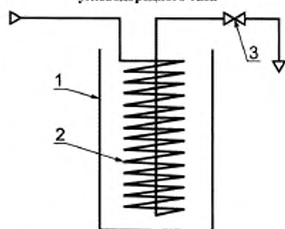
1 — сосуд для охлаждающей смеси; 2 — змеевик; 3 — игольчатый вентиль
