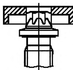
d — Проверка калибром С
