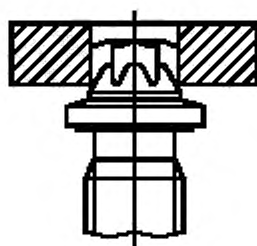
c — Проверка калибром В
