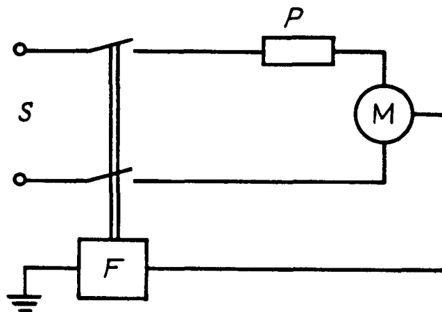
S — сеть питания; М — двигатель вентилятора; Р — защитное устройство (наружное или встроенное); F — прерыватель цепи при токе утечки 30 мА
