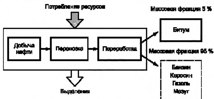
Рисунок 12 — Пример процесса производства битума
