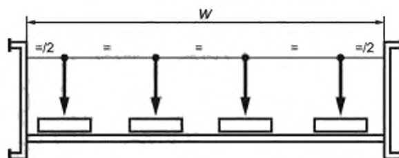
б — точки нагрузки по ширине кабельной лестницы с внешним фланцем
