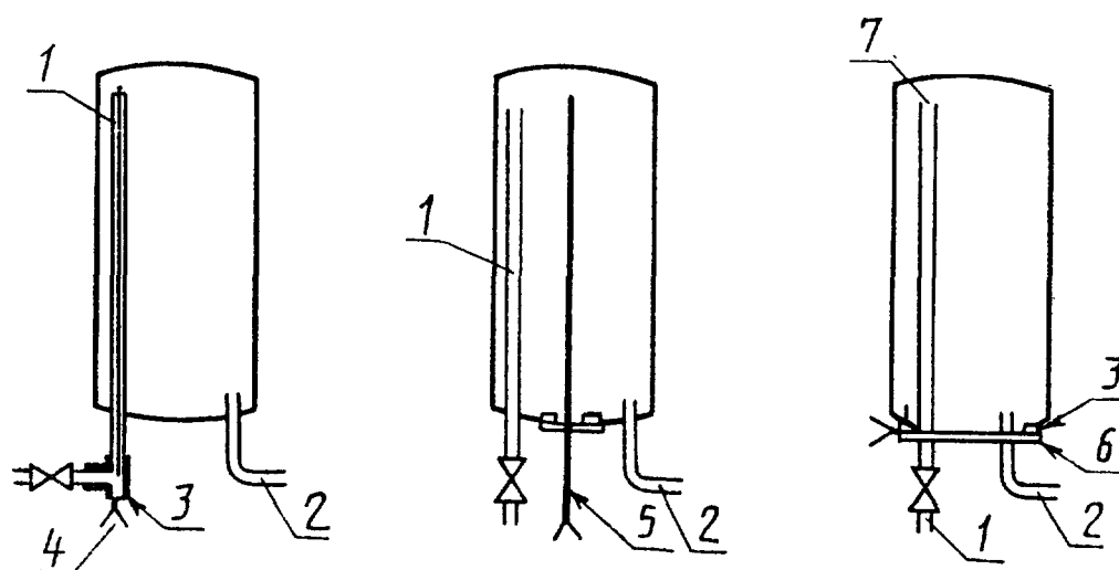
1 — выходная труба; 2 — входная труба; 3 — прокладка; 4 — термопара; 5 — термопара, проходящая через специальную прокладку; 6 — перегородка; 7 — изолированные провода термопары, прикрепленные к выходной трубе и проходящие через специальные прокладки.
