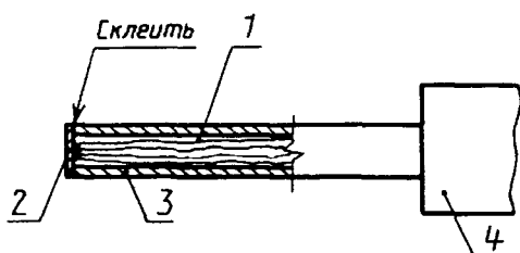
Щуп для измерения температуры поверхности
