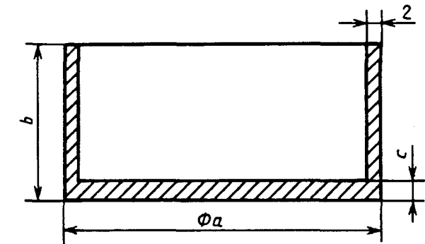
Стандартный испытательный сосуд для нагревательных элементов
