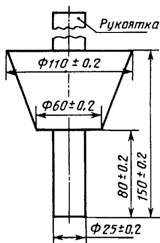
Рисунок 101 — Калибр для проверки измельчителей пищевых отходов
