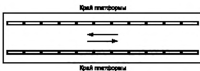
Рисунок А.4 — Форма рифления — одноэлементная тактильная полоса с плоской вершиной (щипиния), используемая для обустройства протяженных предупреждающих ТНУ вдоль края платформ различного назначения
