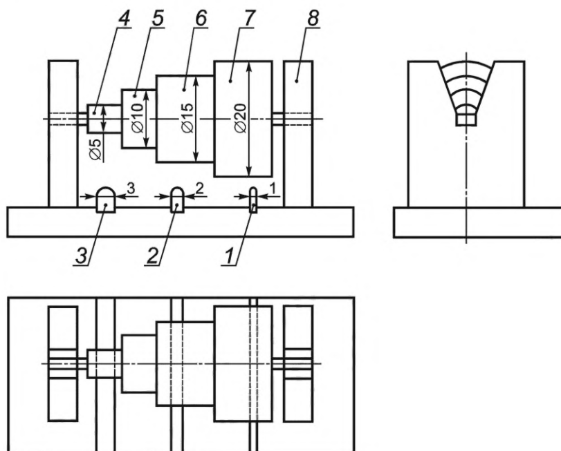
1—7 — стержни; 8 — стойка
