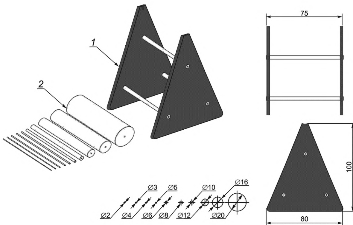
Рисунок А.2 — Устройство прибора типа С
