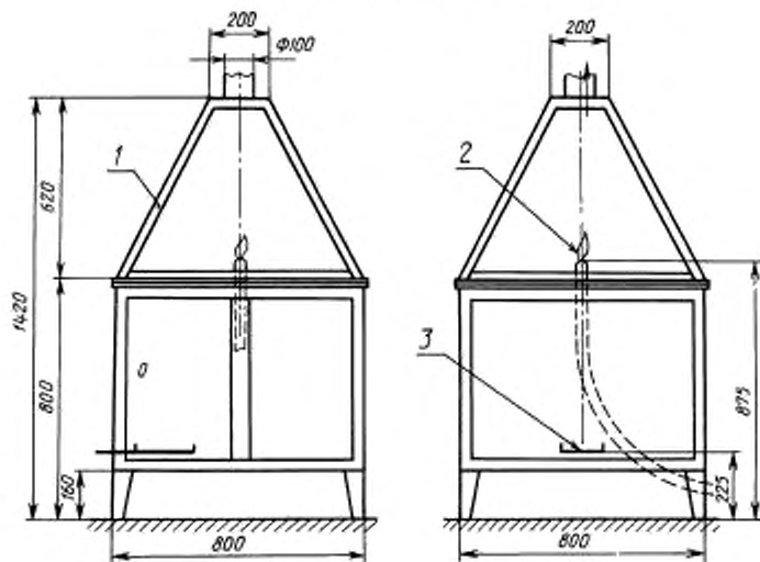
1 — рама из уголка 30×30×3 мм; 2 — механизм зажигания; 3 — поддон-пепельница
