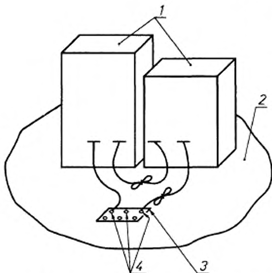
1 — испытуемые ТС; 2 — поворотная платформа; 3 — люк размерами не более (0,1×0,1) м; 4 — розетки сети электропитания (соединительная колодка)
