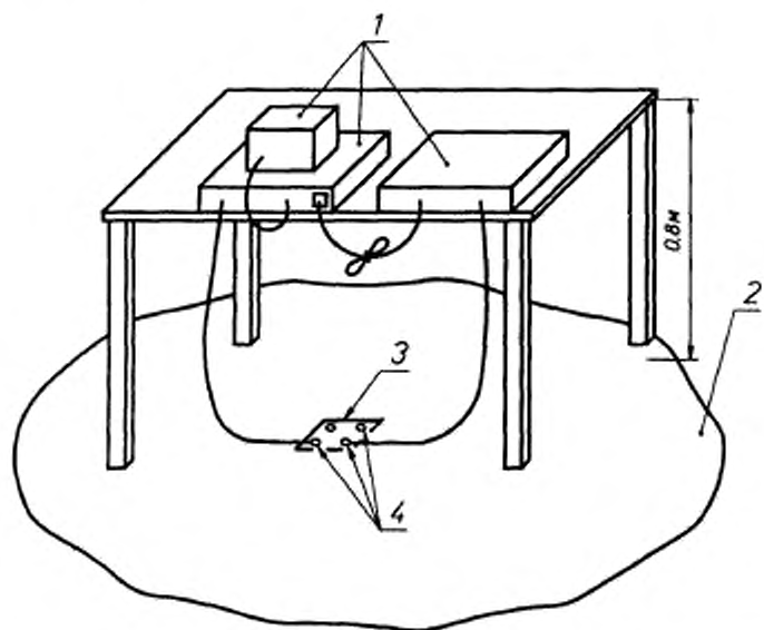
1 — испытуемые ТС; 2 — поворотная платформа; 3 — люк размерами не более (0,1×0,1) м; 4 — розетки сети электропитания (соединительная колодка)
