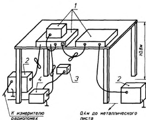
1 — испытуемые ТС; 2 — V-образный эквивалент сети; 3 — имитатор взаимодействующего устройства, подключаемый к зажимам «ЛИНИЯ СВЯЗИ» T-образного эквивалента сети; 4 — T-образный эквивалент сети
