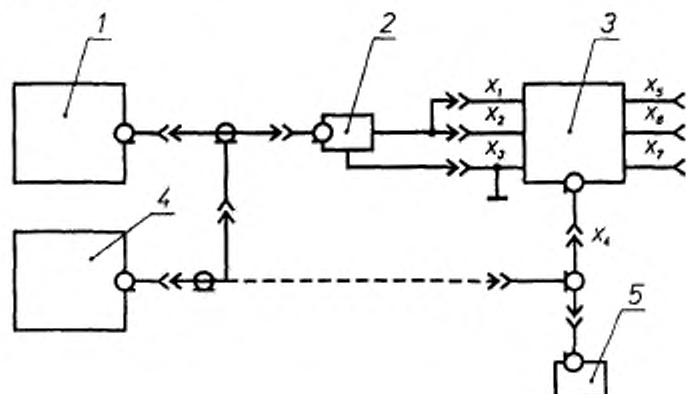
1 — генератор синусоидальных сигналов; 2 — переход, обеспечивающий подключение коаксиального кабеля к зажимам «ИСТОЧНИК РАДИОПОМЕХ» и «ЗЕМЛЯ» Т-образного эквивалента сети; 3 — Т-образный эквивалент сети; 4 — милливольтметр; 5 — эквивалент нагрузки ( Z = 50 \text{ Ом} )
