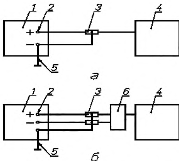
1 — испытуемый объект; 2 — зажим для подключения сети электропитания; 3 — пробник напряжения типа 1; 4 — измеритель радиопомех; 5 — провод заземления (если устройство заземляется); 6 — переключатель фаз; а — однопроводная сеть; б — двухпроводная сеть
