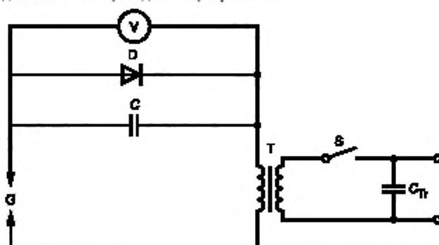
С — основной конденсатор; C_{тр} — конденсатор в цепи триггера; D — диод; S — выключатель; T — трансформатор; G — межэлектродный промежуток; V — импульсный вольтметр
