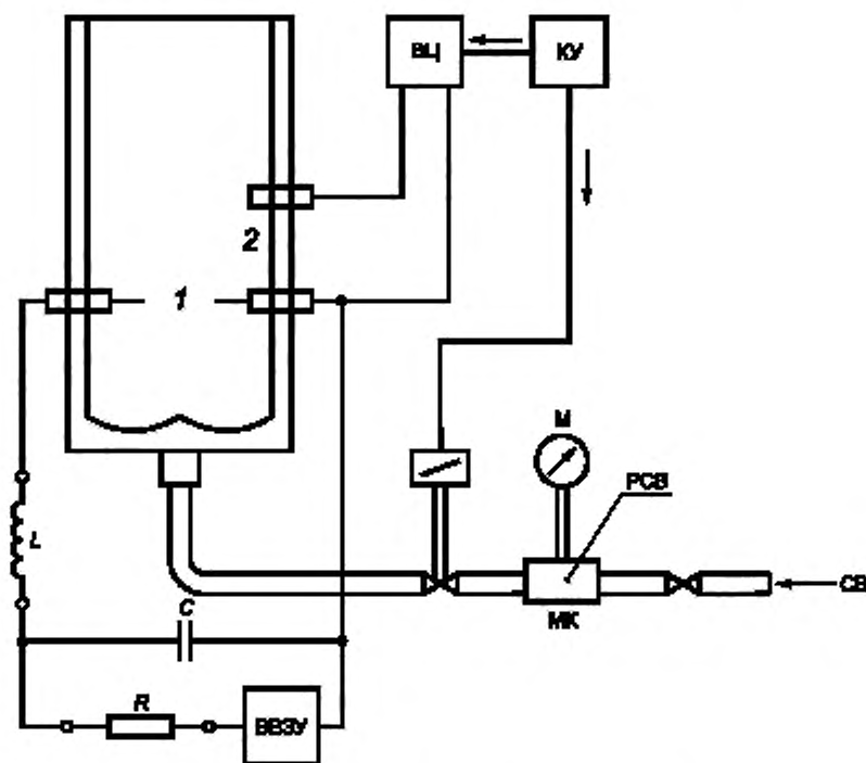
1 — основной межэлектродный промежуток; 2 — вспомогательный электрод; ВЦ — вспомогательная цепь; КУ — контрольное устройство; С — испытательный конденсатор; PCB — резервуар сжатого воздуха; СВ — сжатый воздух; М — манометр; МК — магнитный клапан; К — запорный клапан; ВВЗУ — зарядное устройство; L — индуктивность; R — зарядное сопротивление
