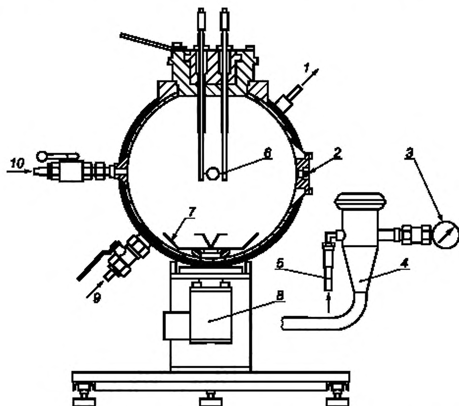
1 -- отверстие для стока воды; 2 -- датчик давления; 3 -- манометр; 4 -- контейнер для пыли (0,6 л); 5 -- впускное отверстие для воздуха; 6 -- источник воспламенения; 7 -- рассеивающая форсунка; 8 -- быстродействующий клапан; 9 -- отверстие для подачи воды; 10 -- выпускное отверстие (воздух, продукты химической реакции)
