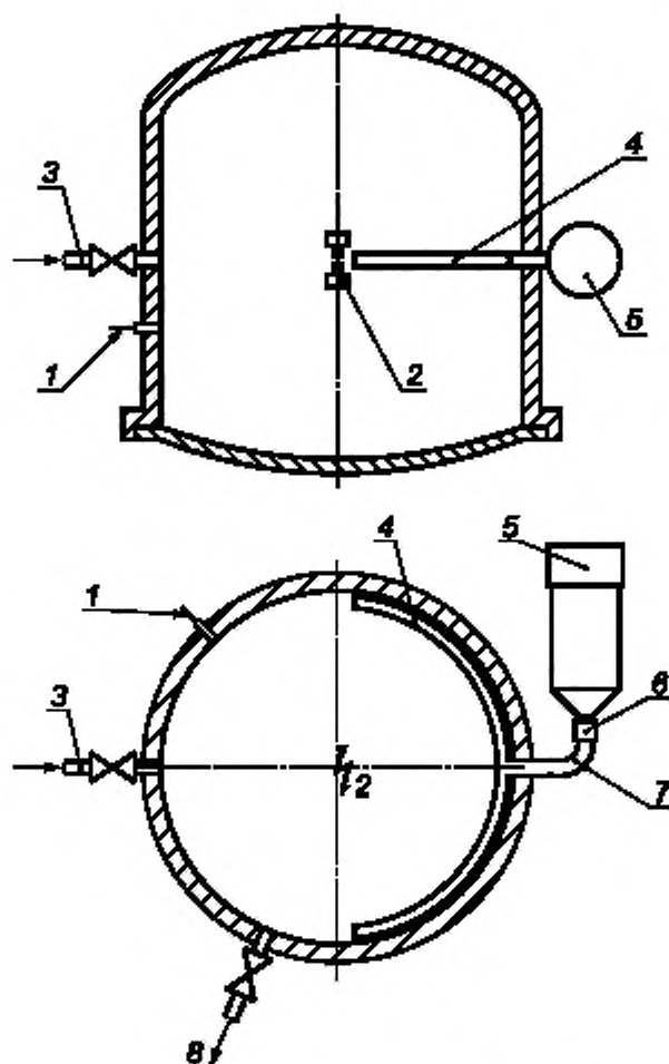
1 — датчик давления; 2 — пиротехнические устройства поджига; 3 — подача продувочного воздуха; 4 — полукруглое раздаточное устройство; 5 — контейнер для пыли; 6 — быстродействующий клапан; 7 — соединительная трубка; 8 — выходное отверстие для удаления газа
