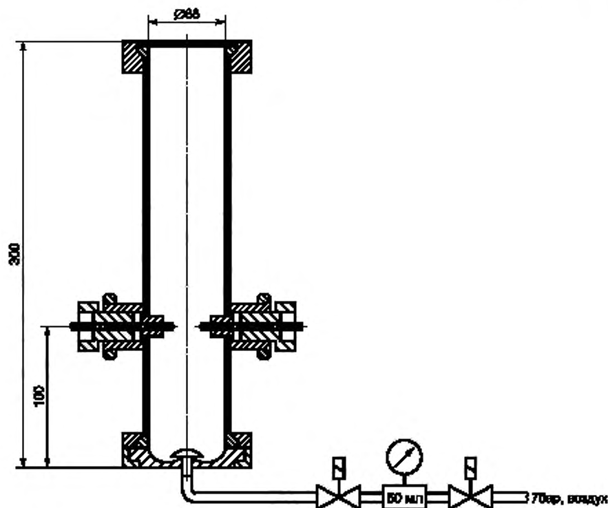
Рисунок 4 — Модифицированная трубка Гартмана
