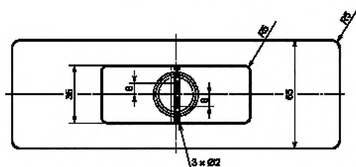
Рисунок Е.3 — Вид сверху рассеивающей форсунки
