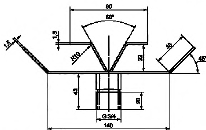
Рисунок Е.2 — Изображение поперечного сечения рассеивающей форсунки
