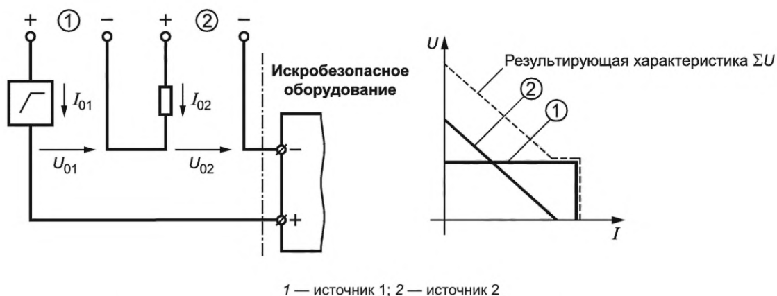
а) — Последовательное подключение со сложением значений напряжения
