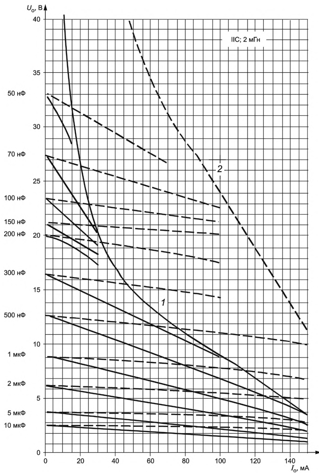
d) Диаграмма для значения 2 мГц
