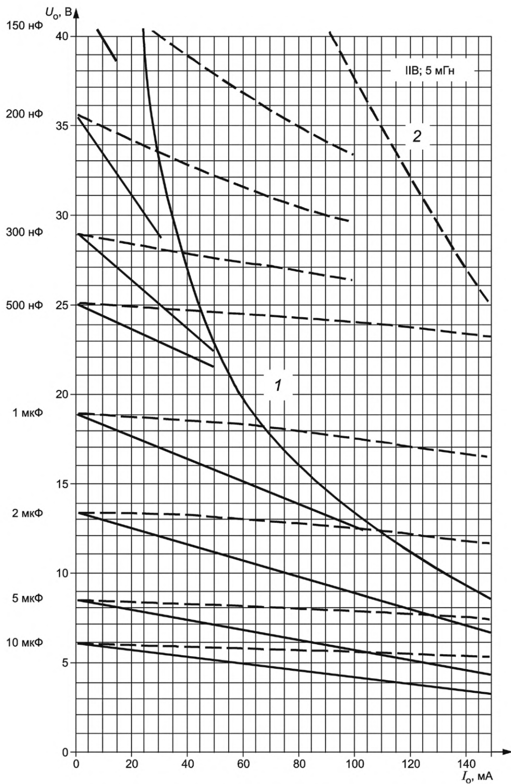
е) Диаграмма для значения 5 мГн
