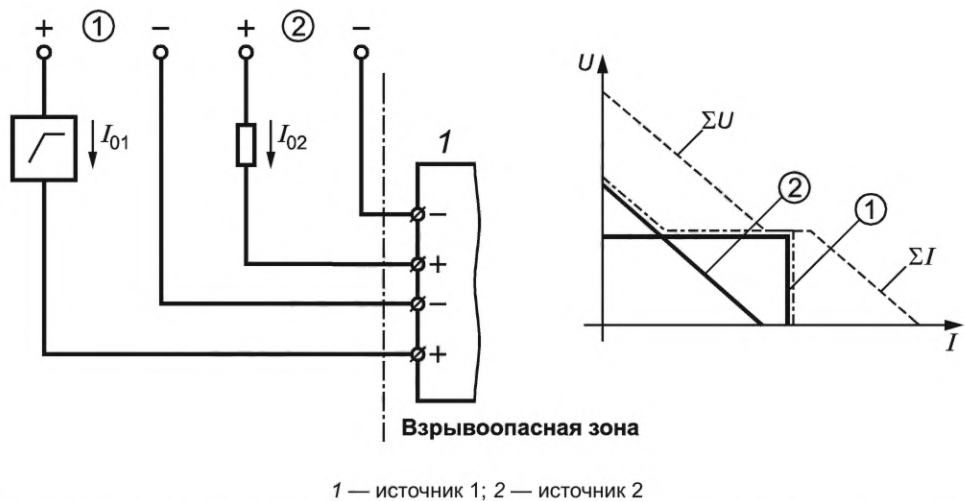
е) — Последовательное или параллельное подключение со сложением значений тока и напряжения
