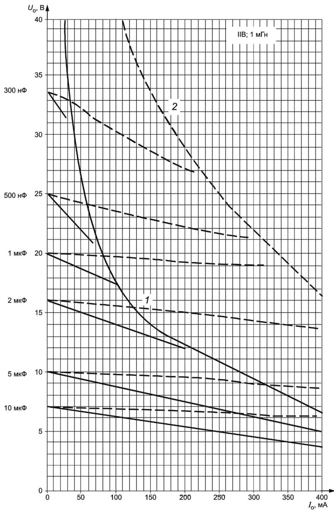
с) Диаграмма для значения 1 мГн
