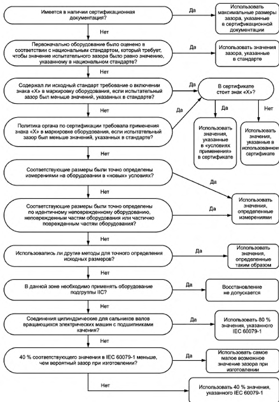
Рисунок С.1 — Определение максимального зазора для восстановленных деталей
