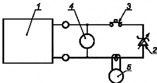
1 — испытываемая цепь; 2 — нагрузка; 3 — плавкий выключатель; 4 — вольтметр высокого сопротивления; 5 — шуп для замера величины тока
