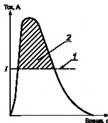
1 — ток I , максимально допустимый в соответствии с испытанием на искробезопасность или оценкой по приложению А; 2 — передаваемая энергия (Дж) — напряжение V(B) × заштрихованный участок кривой (А.с)
