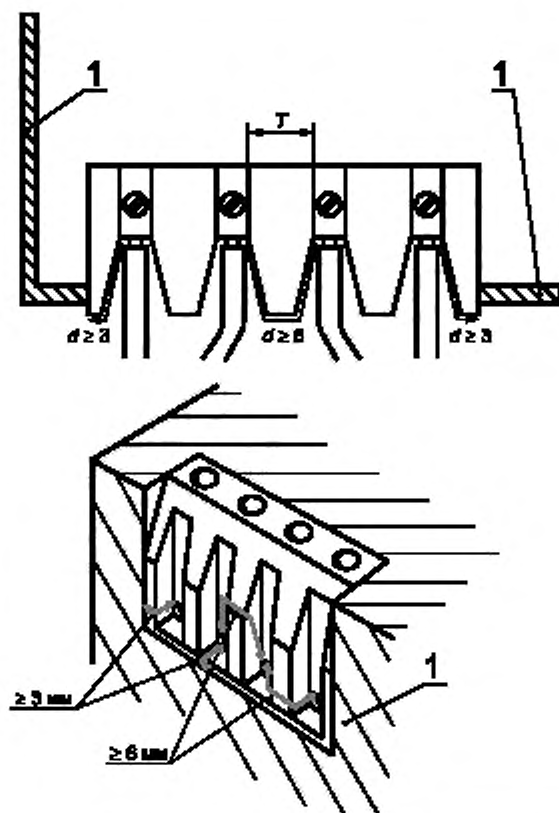
1 — токопроводящая часть, T — электрические зазоры и длина путей утечки в соответствии с 6.3, d — электрические зазоры на внешних соединительных устройствах зажимов в соответствии с 6.2.1
