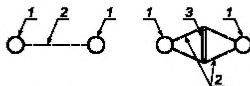
1 — проводник; 2 — электрический зазор; 3 — перегородка
