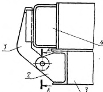
1—кронштейн; 2—проушина; 3—поддон; 4—борт
