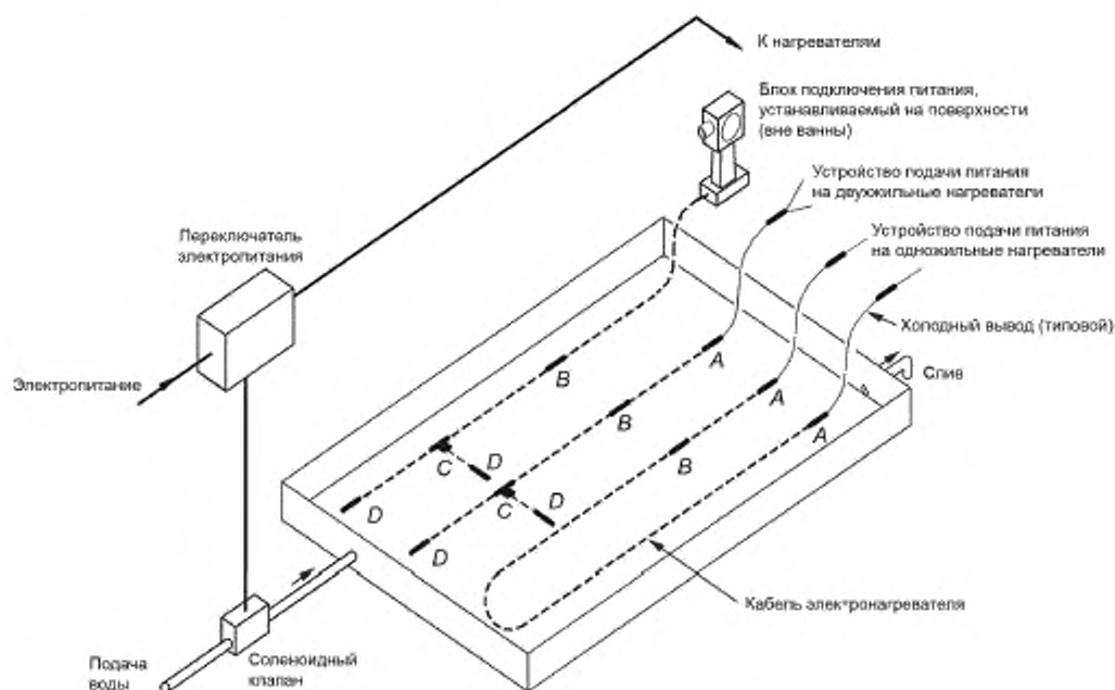
А — встроенный силовой соединитель, В — встроенный соединитель нагревательного элемента, С — встроенный Т-образный соединитель; D — встроенный концевой соединитель
