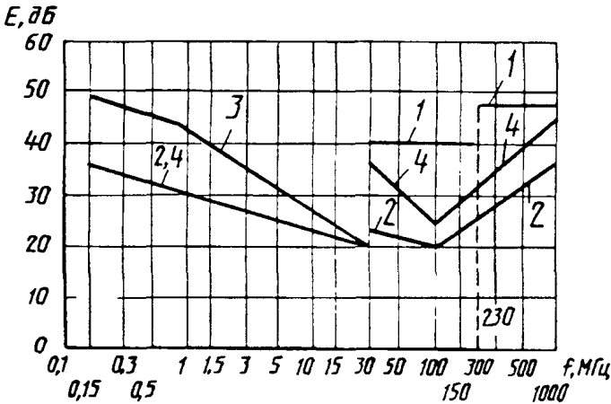
Нормы напряженности поля радиопомех
