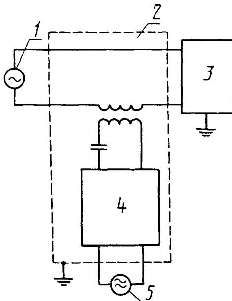
1 — источник питания; 2 — ИГ; 3 — ИТС; 4 — усилитель мощности гармоник; 5 — источник напряжения гармоник
