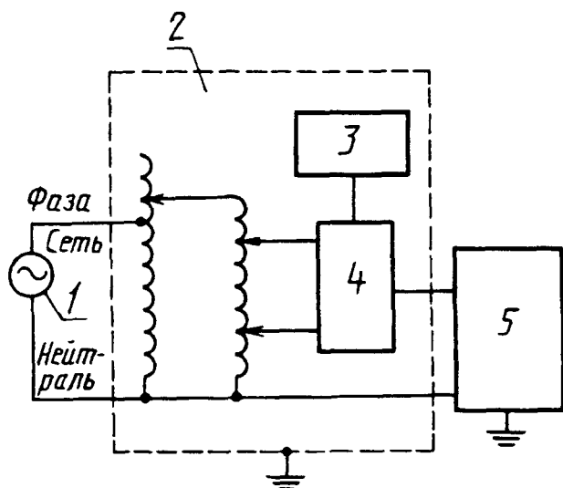
1 — источник питания; 2 — ИГ; 3 — блок управления; 4 — блок коммутации; 5 — ИТС
