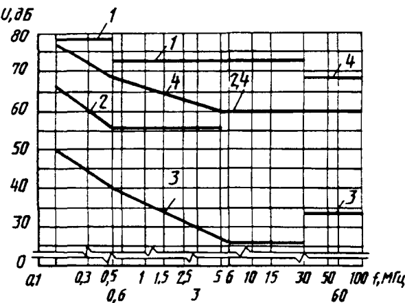
Нормы напряжения радиопомех
