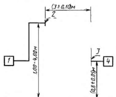
1 — ВЧ генератор; 2 — излучающая антенна; 3 — приемная антенна; 4 — измерительный приемник
