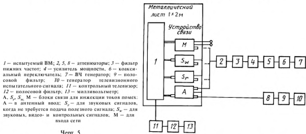
Схема расположения аппаратуры при испытаниях на устойчивость ВМ к наведенным ВЧ токам
