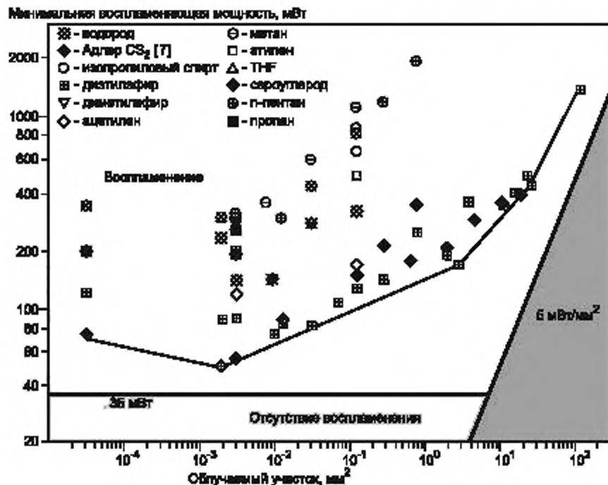
Рисунок В.1 — Минимальная воспламеняющая мощность излучения с инертным поглотителем в качестве облучаемого материала ( \alpha \cdot 0.04 \text{ мм} = 83\% , \alpha \cdot 0.05 \text{ мм} = 93 ) при непрерывном облучении в волновом диапазоне 1064 нм
