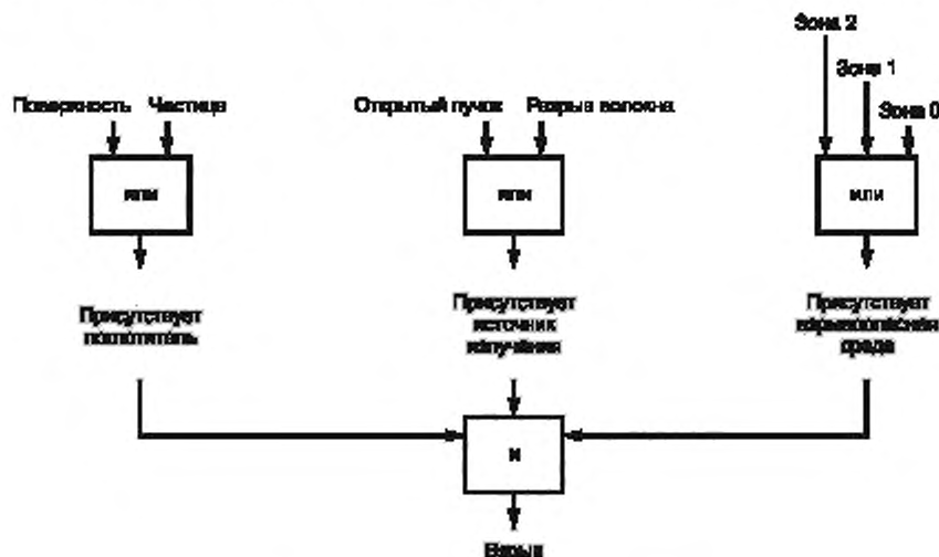
Рисунок С.1 — Оценка опасности воспламенения
