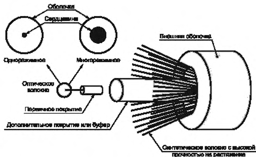
Рисунок D.2 — Типовая конструкция одноволоконного оптического волокна
