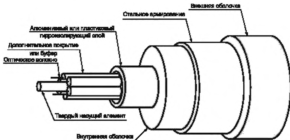
Рисунок D.1 — Пример конструкции многоволоконного оптического кабеля для эксплуатации в тяжелых условиях
