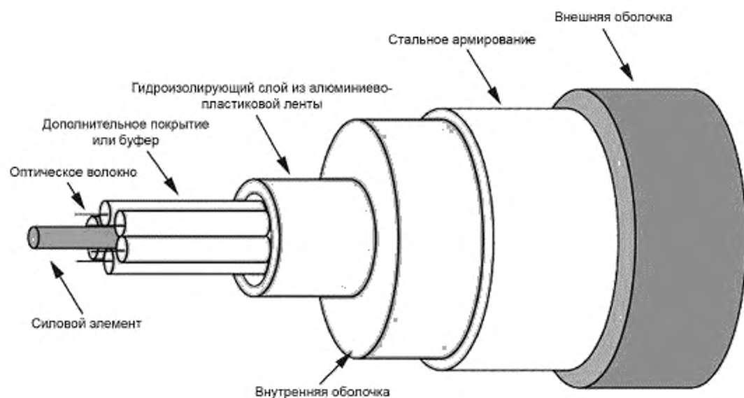
Рисунок D.1 — Пример конструкции многоволоконного оптического кабеля для эксплуатации в тяжелых условиях
