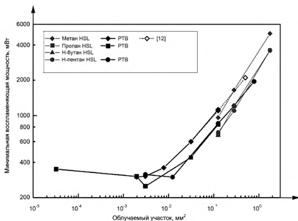
Рисунок В.2 — Минимальная воспламеняющая мощность излучения с инертным поглотителем в качестве облучаемого материала ( \alpha_{1064 \text{ нм}} = 83 \% , \alpha_{805 \text{ нм}} = 93 \% ) при непрерывном облучении (PTB: 1064 нм, HSL: 805 нм [12]: 803 нм) для некоторых n-алканов
