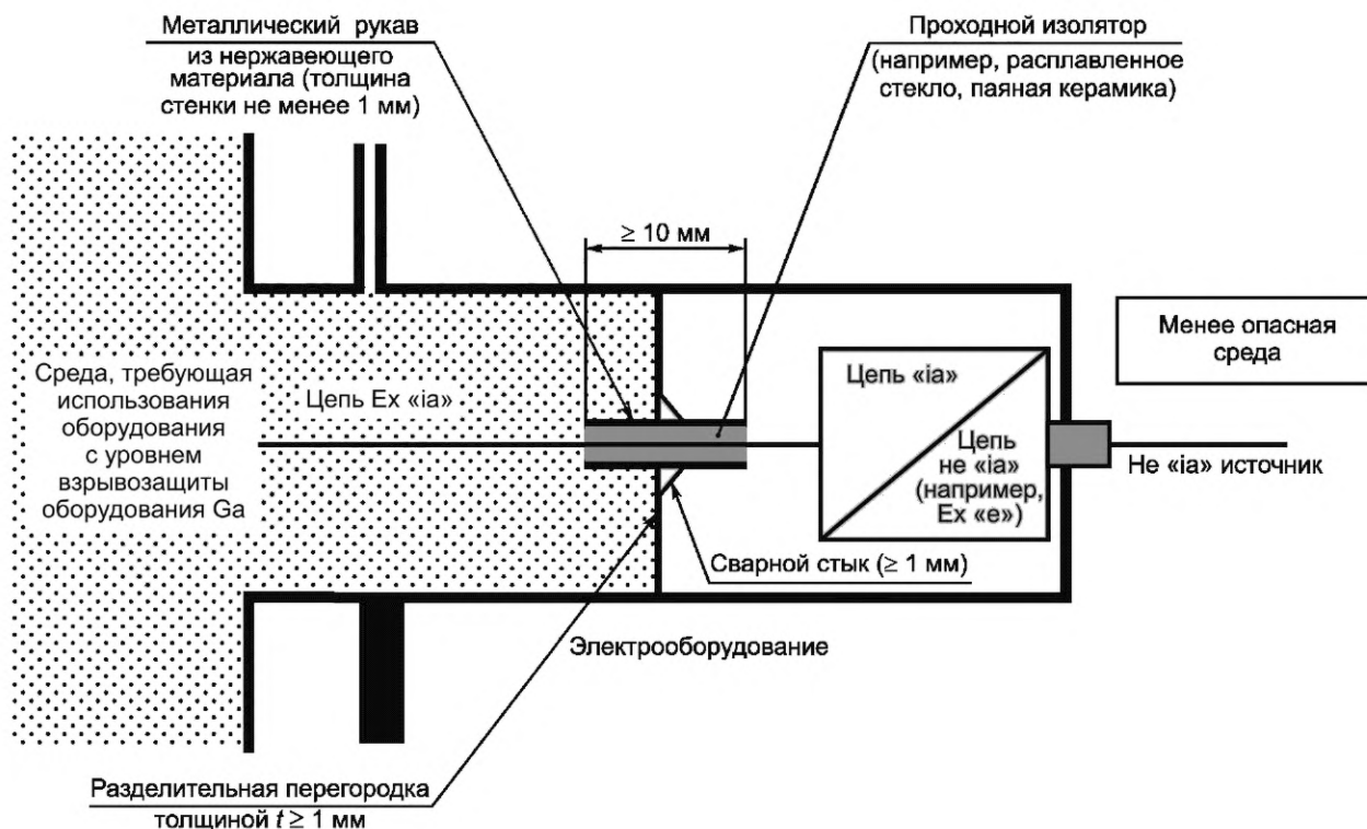
Рисунок 1 — Пример газонепроницаемой разделительной перегородки с проходным изолятором
