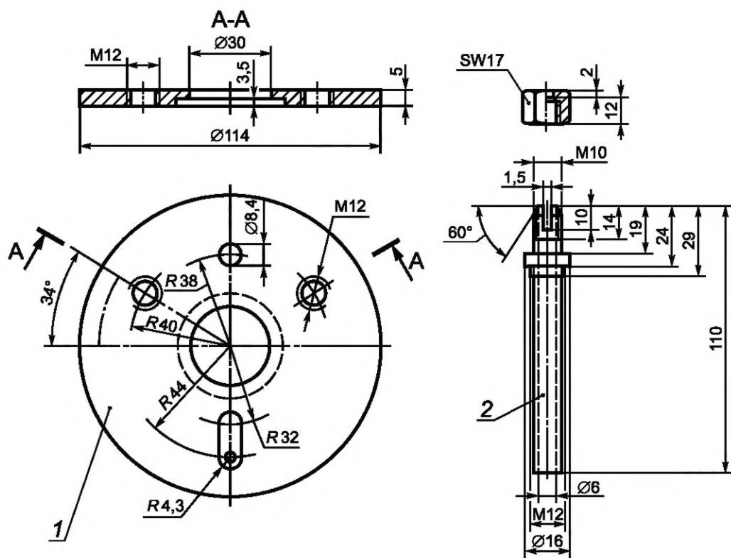
Рисунок А.7 — Крышка стального цилиндра
