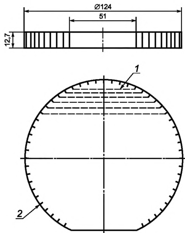
1 — способ укладки никель-хромового провода диаметром 0,4 мм и длиной 2,5 м; 2 — паз размером 1,5×1,5 мм на боковой поверхности диска
