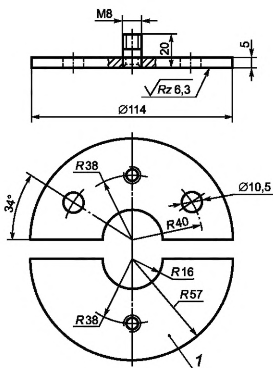
Рисунок А.7 — Крышка стального цилиндра
