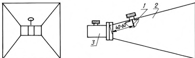
Приемопередающая антенна
