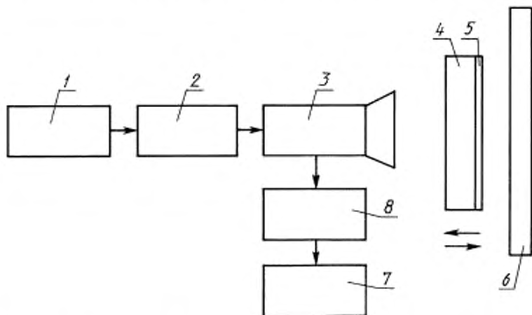
1 — генератор; 2 — вентиль или аттенюатор; 3 — антенна приемопередающая; 4 — испытуемый образец ПЭВ; 5 — металлический лист; 6 — экран из ПЭВ; 7 — усилитель селективный; 8 — детекторная головка с зондом
