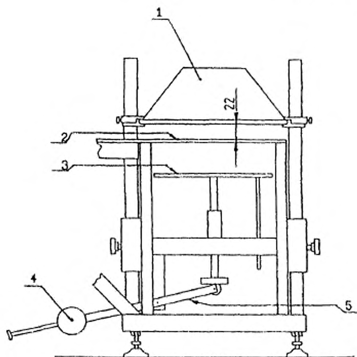
1 — радиационная панель; 2 — защитная плита, 3 — подвижная платформа; 4 — протирок; 5 — рычаг
