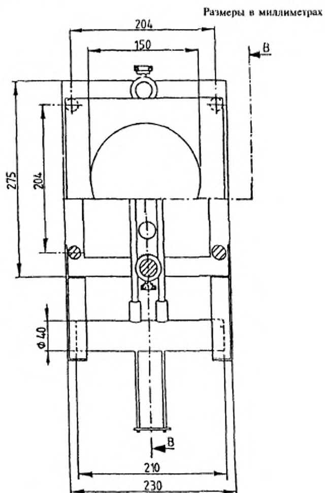
Рисунок А3 — Опорная станина (разрез по АА)
