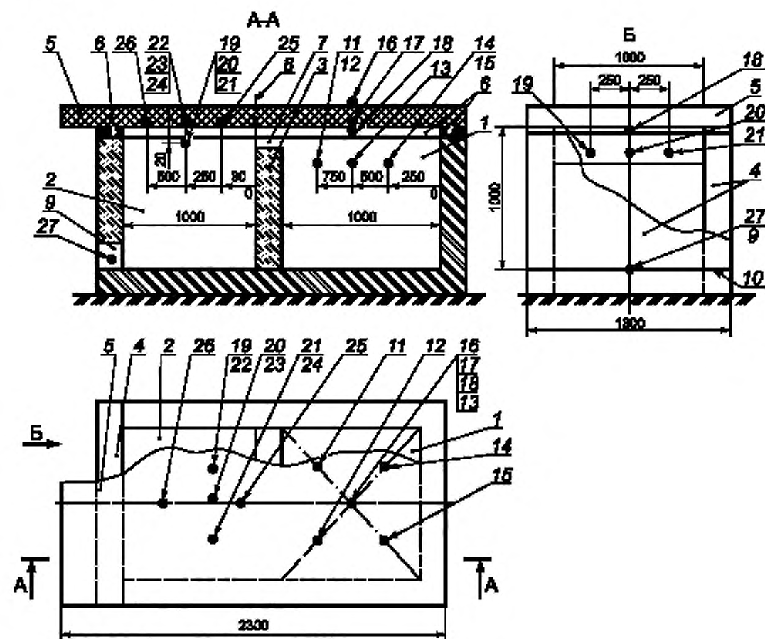
1 — огневая камера; 2 — тепловая камера; 3 — перегородка, разделяющая огневую и тепловую камеры; 4 — ограждение тепловой камеры; 5 — образец; 6 — уплотнение; 7 — проем между обогреваемой поверхностью образца и торцом перегородки 3; 8 — граница тепловой камеры и контрольной зоны образца; 9 — проем для выходов газа; 10 — прокладка; 11—27 — термопары для измерения температуры конструкции и газовой среды в огневой и тепловой камерах
