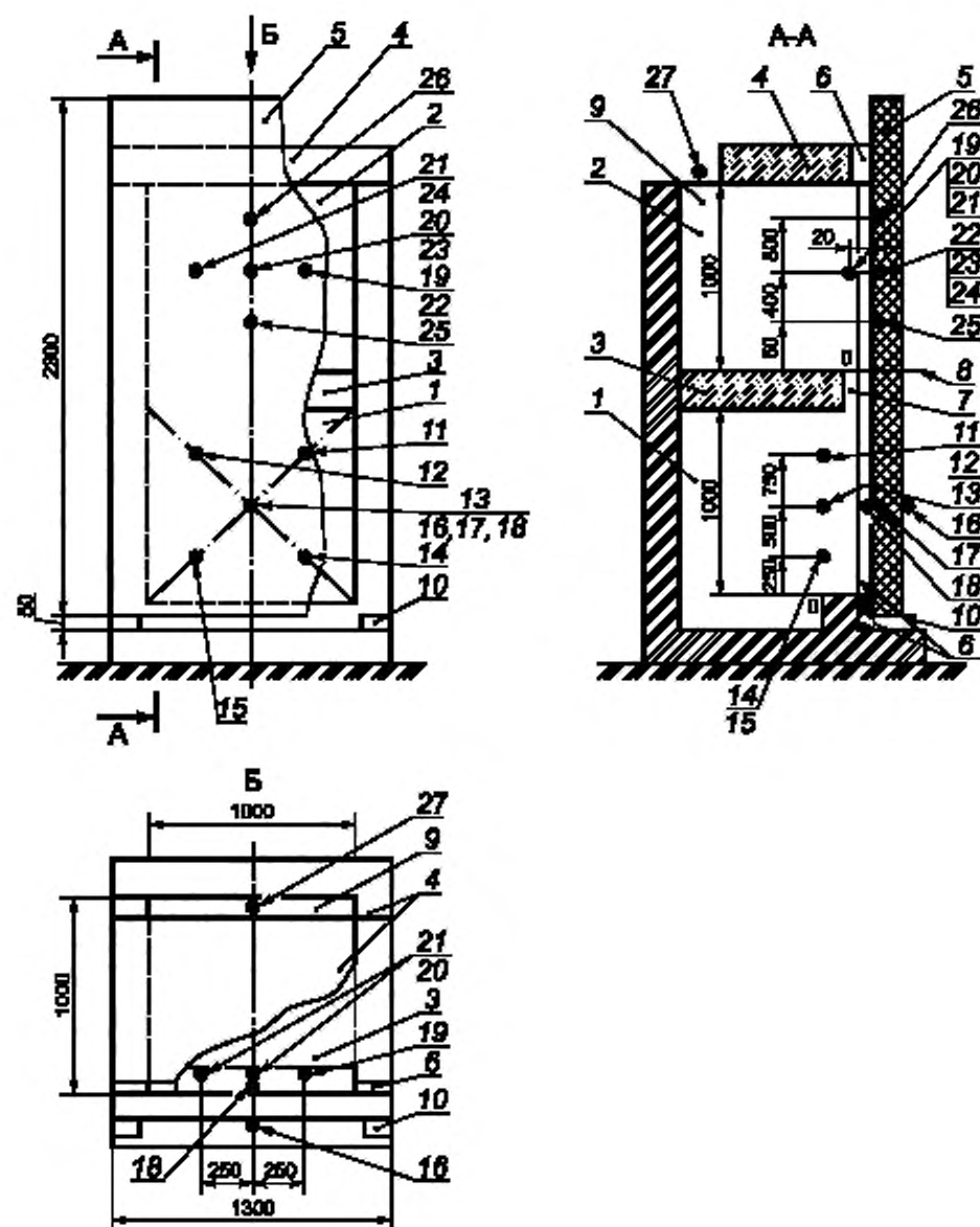
1 — огневая камера; 2 — тепловая камера; 3 — перегородка, разделяющая огневую и тепловую камеры; 4 — ограждение тепловой камеры; 5 — образец; 6 — уплотнение; 7 — проем между обогреваемой поверхностью образца и торцом перегородки 3; 8 — граница тепловой камеры и контрольной зоны образца; 9 — проем для выходов газа; 10 — прокладка; 11—27 — термопары для измерения температуры конструкции и газовой среды в огневой и тепловой камерах
