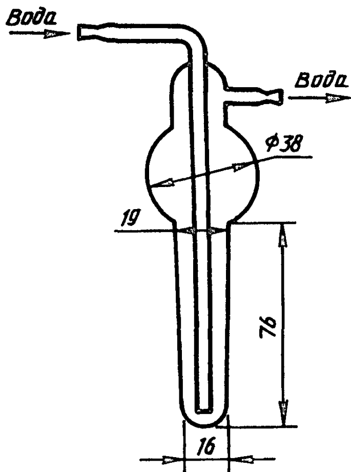
Рисунок 1 — Штифтовый холодильник
