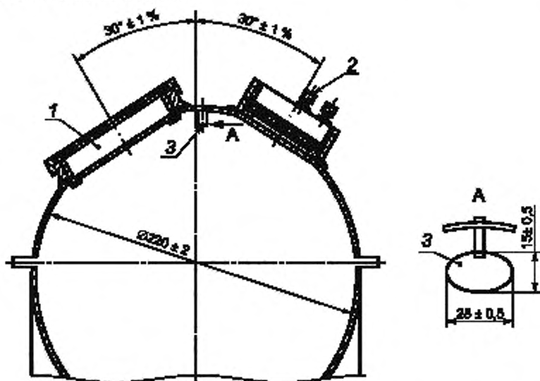
Рисунок А.1 — Схема светомерного шара
