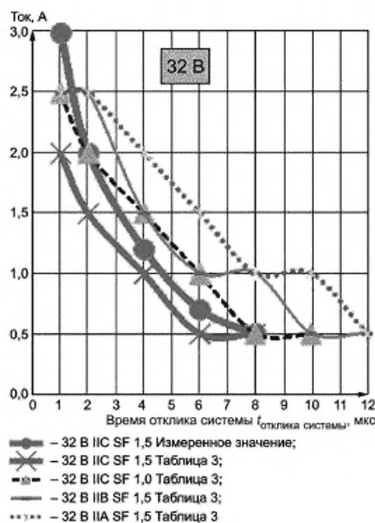
Рисунок В.9 — Значения воспламенения Power-i для класса напряжения 32 В (32 В постоянного тока)
