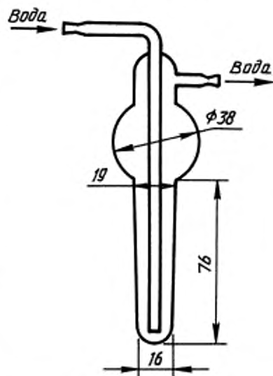
Рисунок 2 — Пальчиковый холодильник
