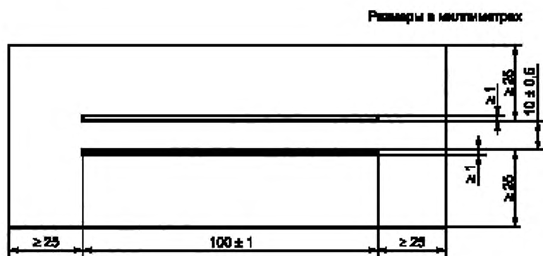
Рисунок G.1 — Испытуемый образец с установленными электродами
