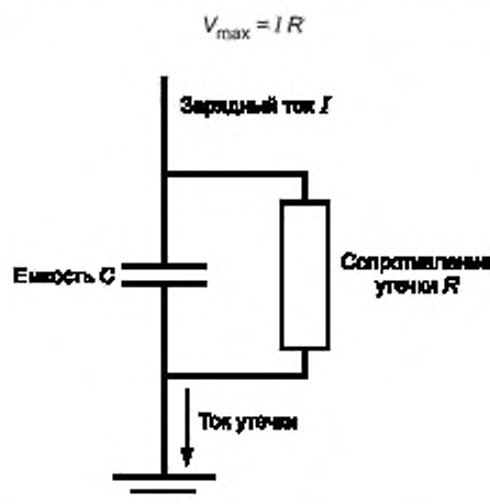
Рисунок А.1 — Эквивалентная электрическая цепь электростатического заряжения проводника
