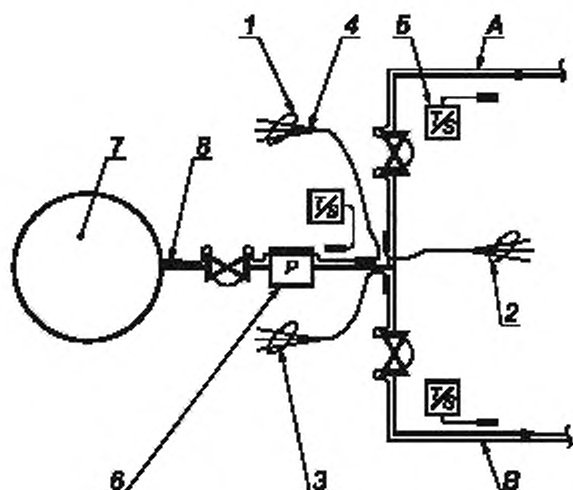
А — труба А; 1 — цепь № 1; 2 — цепь № 2; 3 — цепь № 3; 4 — заделка холодного конца; В — труба В; 5 — температурный датчик; 6 — насос; 7 — обогреваемый резервуар; 8 — заделка горячего конца
