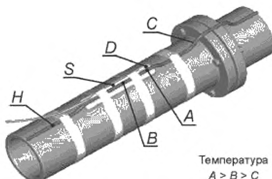
H — электронагреватель; S — датчик температуры; A — температура искусственного горячего пятна; B — температура в точке измерения; C — точка с плохим тепловым сопряжением (типичное горячее пятно); D — теплоизоляция между электронагревателем и нагретой поверхностью
