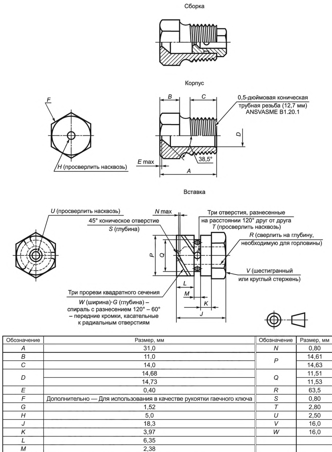
Рисунок В.2 — Распылительная головка
