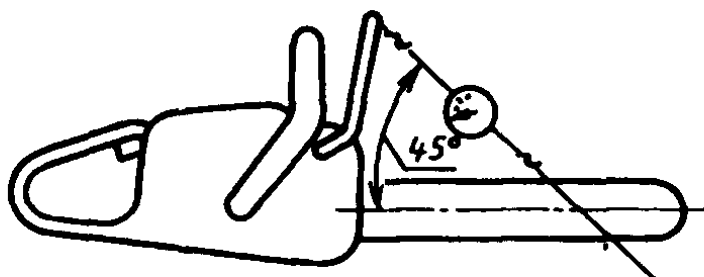
Рисунок 1 — Статическое испытание силы размыкания тормоза
